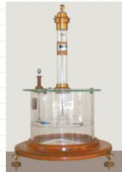
Bilancia a torsione per la verifica della legge di Coulomb
